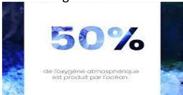
Oxygène
