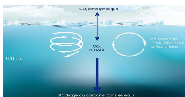
CO2
